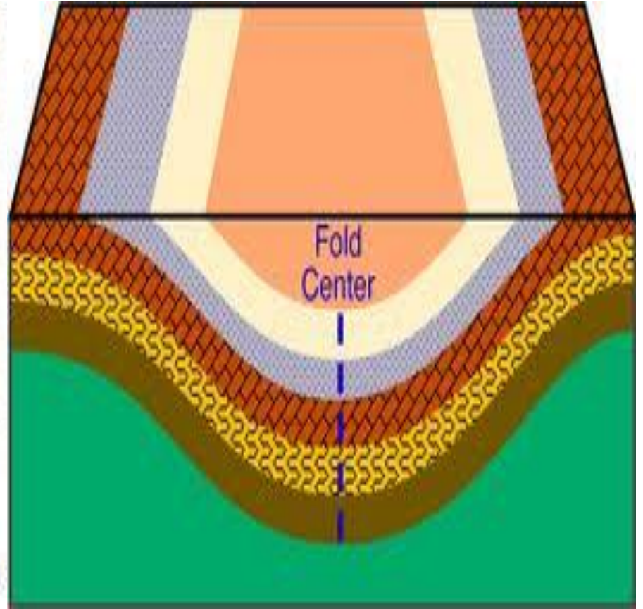
منظر جيولوجي بمنطقة الريش يبين طية مقعرة الطبقة a أحدث من الطبقتين b و c.
