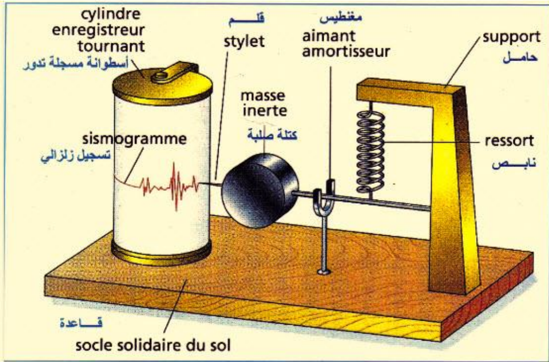
SISMOMETRE CLASSIQUE مسجل الزلازل الكلاسيكي
